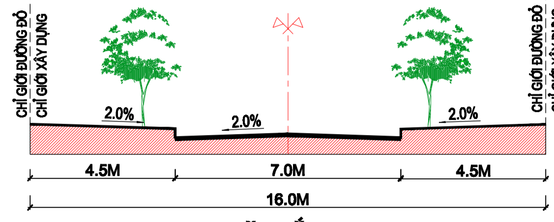
MẶT CẮT 2-2
