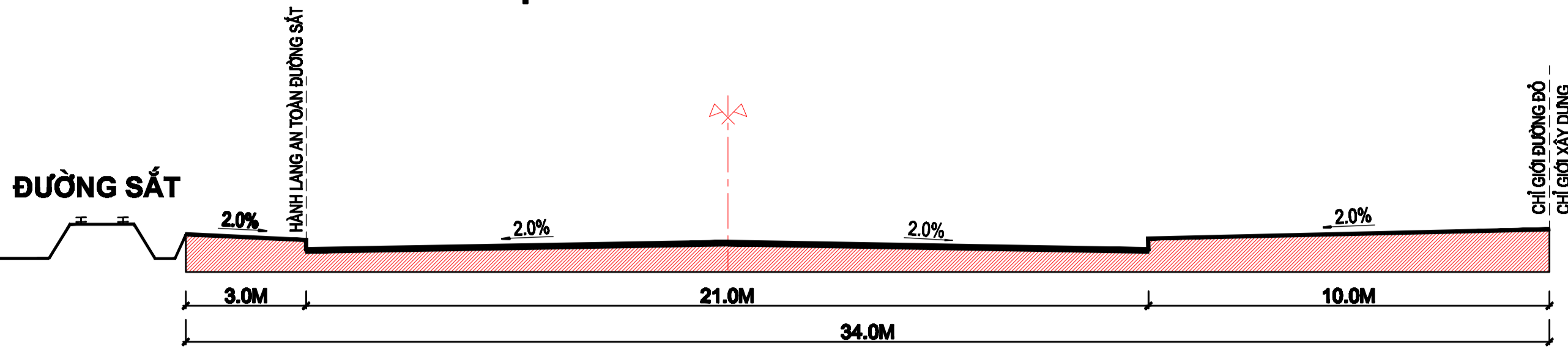
MẶT CẮT 1-1
